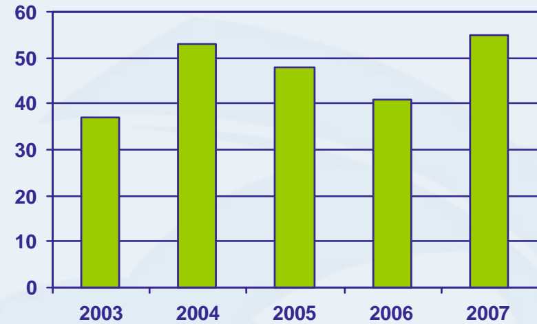
IPv6 - Prefixes
